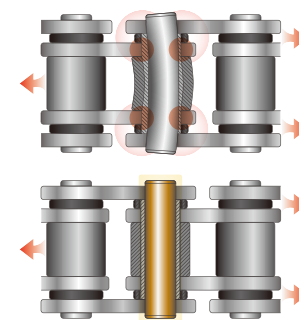
赛车激烈加速和刹车时，对链条冲击力极大。高强度的销轴可满足这一要求。
