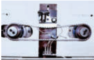
回转疲劳试验机 Rotary Fatigue Testing Machine 设备作用： 检测链条回转疲劳性能 Detect the chain rotary fatigue performance
